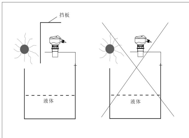
图 35 温度变化大--加遮阳板或者仪表箱
