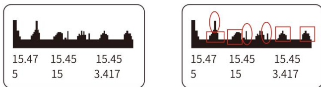
图 53 变频器干扰的回波图形
