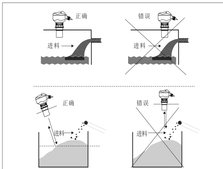
图 29 传感器不要安装在进料的料流里或者上方
