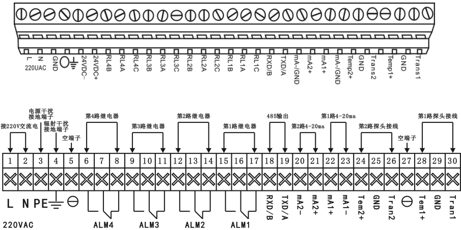
图 36 电气连接图和接线端子示意图
