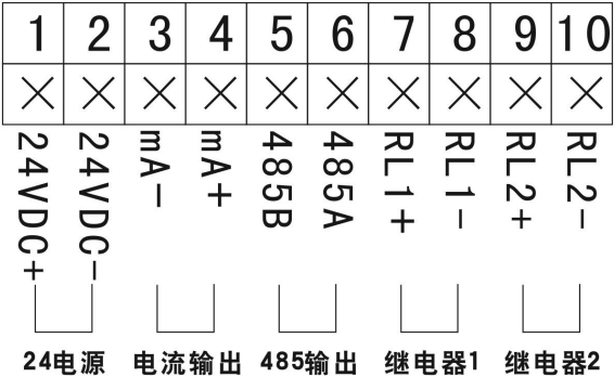
图 40 四线制 24VDC 供电接线图
