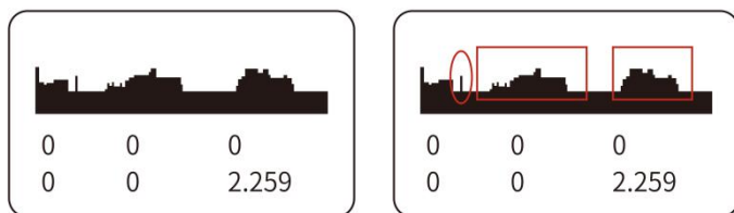
图 52 变频器干扰的回波图形
