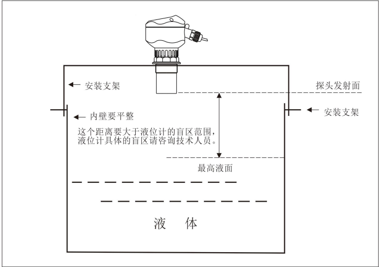
图 16 开口容器上--顶部居中支架安装
