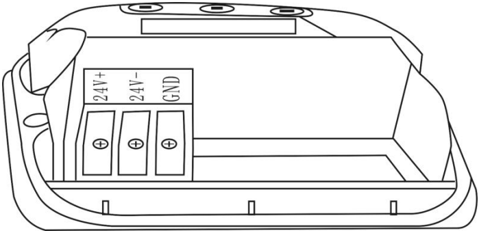
图 42 二线制电气连接图
