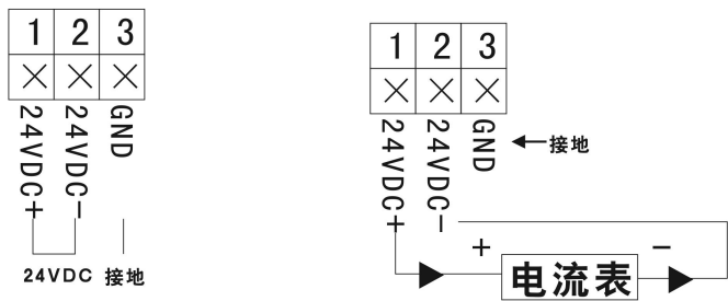
图 43 二线制接线示意图和二线制接电流表示意图
