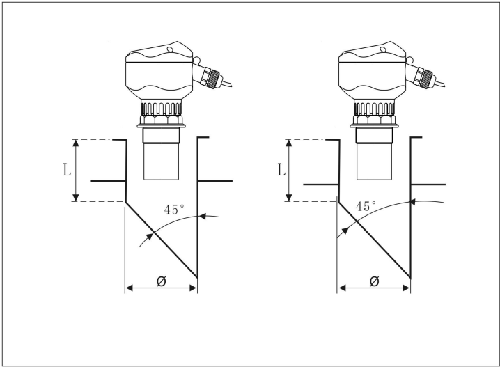
图 24 不浸泡在介质中的延长接管
