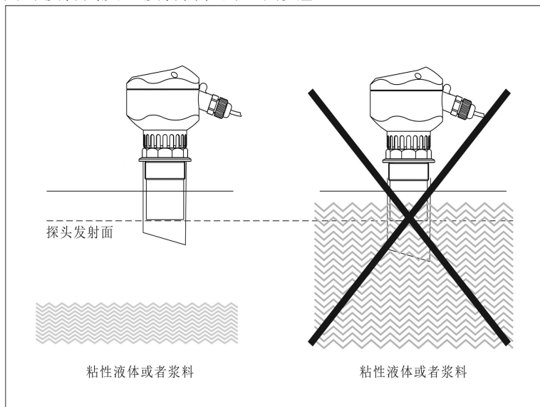
图 23 接管不能浸泡在粘附性介质里
