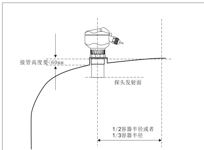
图 13 安装在螺纹接管上--拱形罐顶
