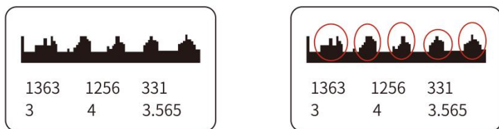
图 51 变频器干扰的回波图形
