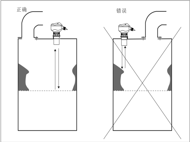
图 30 容器壁有粘附物--要距离粘附物一定距离
