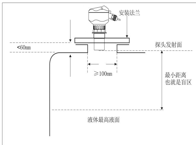
图 8 法兰安装，安装在很短的接管内
