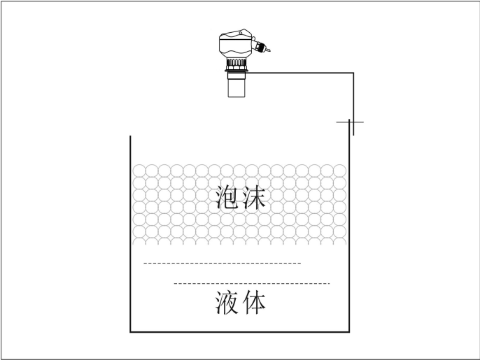
图 33 产生气泡的场合
