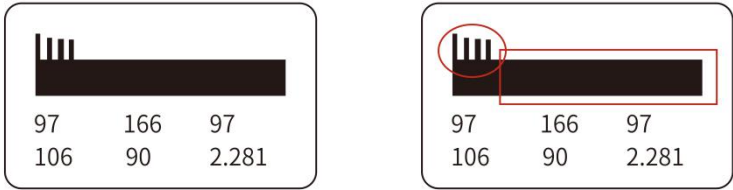
图 55 探头缩在接管内的回波
