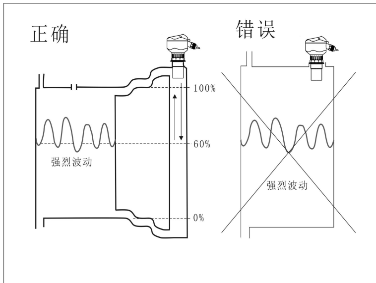
图 32 介质表面波动大--用旁通管或者加导波管测量
