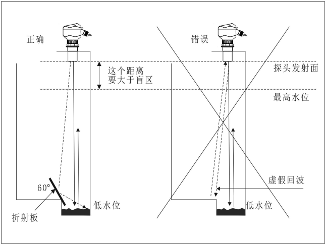
图 31 水池底部有障碍物--用挡板折射走
