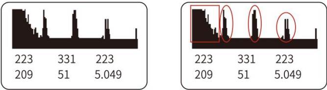
图 45 共振形成的回波信号
