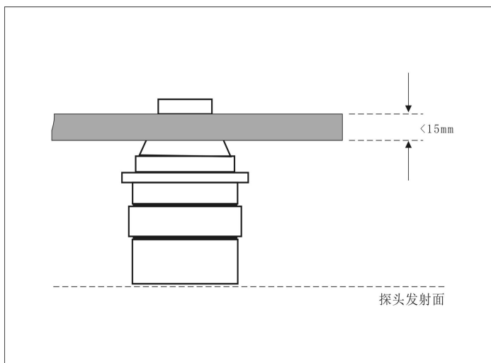
图 12 分体式探头顶吊螺纹连接
