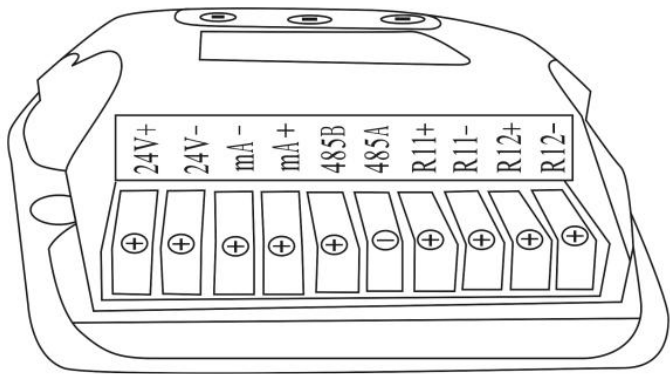
图 39 一体式增强型四线制电气连接图
