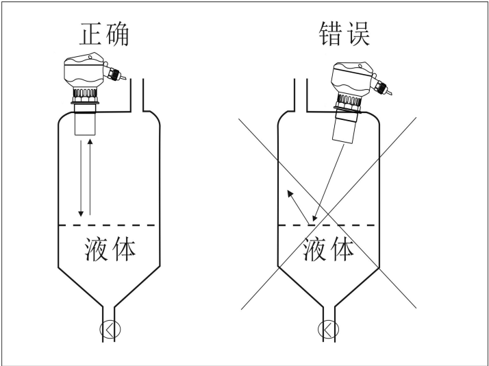
图 34 传感器探头应垂直于介质表面
