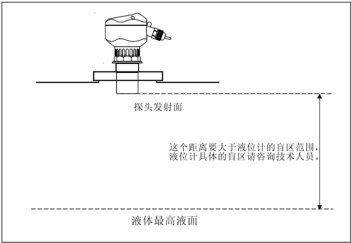
图 10 法兰型安装在无接管平顶罐上
