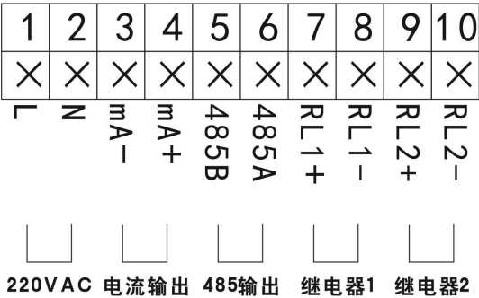
图 41 四线制 220VAC 电气连接图
