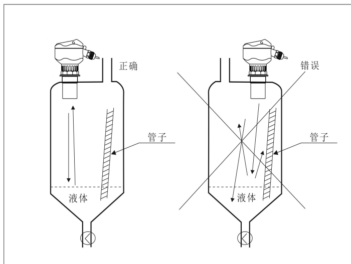
图 28 容器内的障碍物--管子
