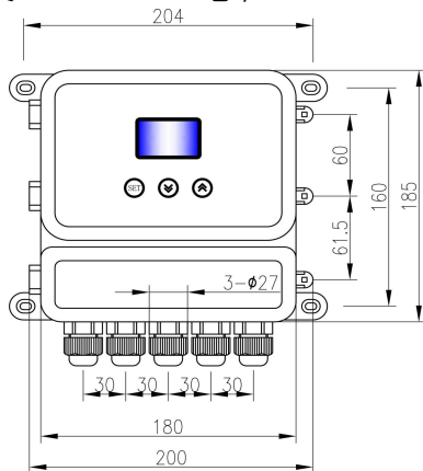
图3 分体式结构图
